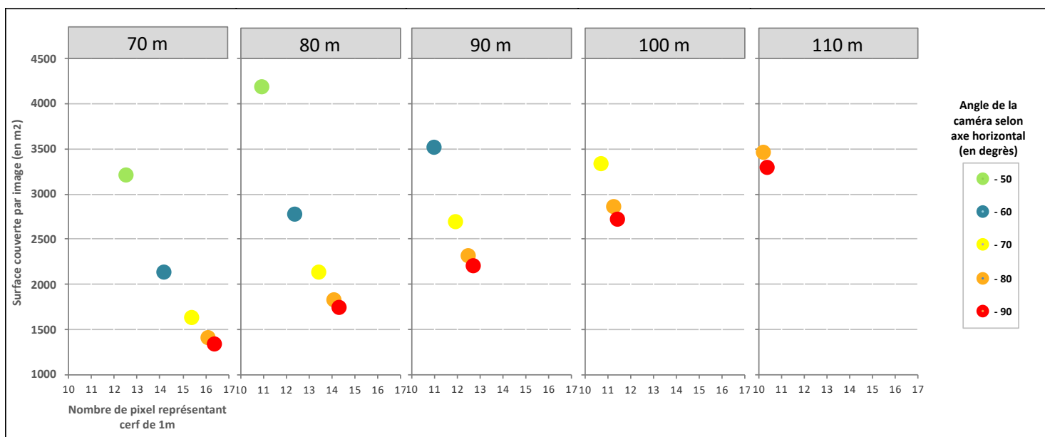
Figure 16 : Graphiques représentant, selon l'angle de caméra (de -50 à -90 °) et la hauteur du drone (70 à 110 m), le nombre de pixel structurant un cerf de 1 m de long et la superficie (en m 2 ) couverte par l'image.
