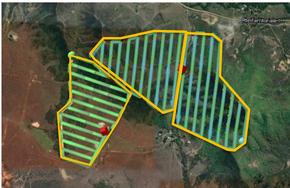
Figure 25 : Ensemble des missions drones avec capteur thermique réalisées au cours de l'étude en mode balayage de zone et suivi de terrain sur la propriété de la ferme de chasse La Cotonnière (Boulouparis).
