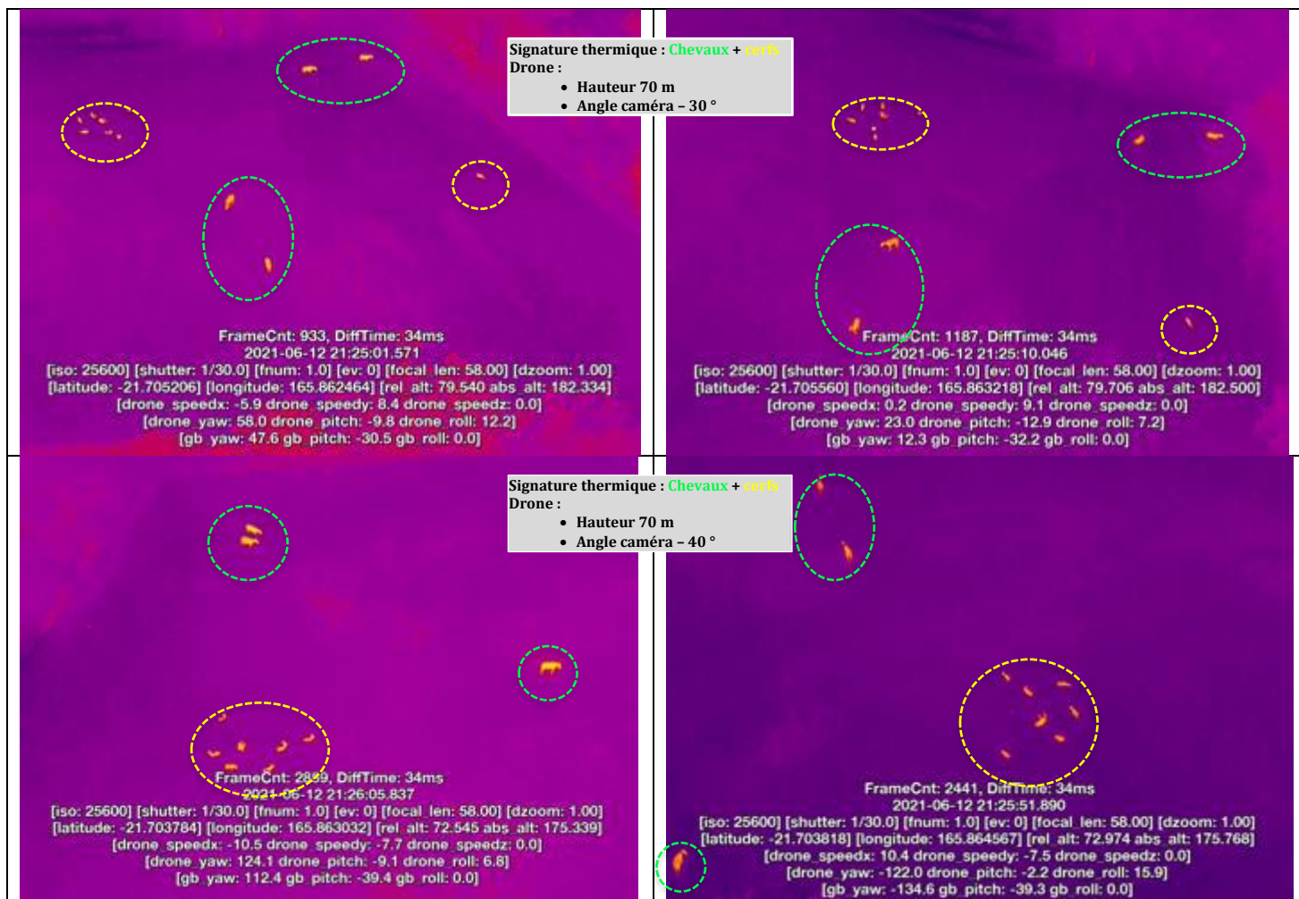
Planche photos 3 : Observation des différences de signatures thermiques de nuit par drone thermique entre cheval et cerfs à hauteur de vol et angle caméra similaires.
