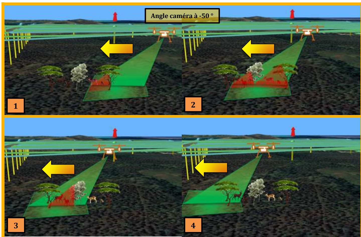
Figure 34 : Simulation des empreintes au sol lors d'un passage du drone dans de la végétation arborée avec des animaux (cerfs) pour un angle caméra de -50^\circ et une hauteur de vol de 70 m. En rouge est représenté l'angle de vue avec des animaux (ou partie d'animaux) caché par cette végétation.
