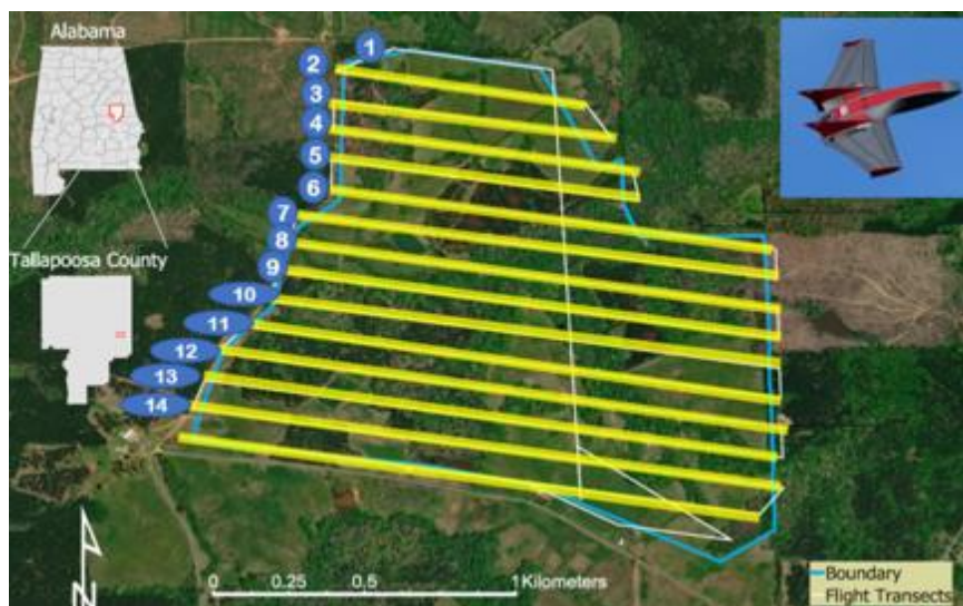
Figure 6 : Exemple de Trajectoire de vol (lignes blanches) en blocs (balayage de zone en forme de polygone) et transects parcourus (surlignés en jaune et étiquetés) tiré de l'étude de Beaver et al. 2020 pour des relevés thermiques par drones sur le cerf de Virginie
